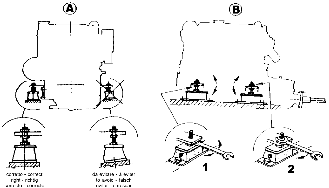
schema di montaggio dei supporti antivibranti - Schéma de montages des supports anti-vibration Silent blocks assembly diagram - Montageschema der schwingungsdämpfenden Halterung Esquema de montaje de los soportes antivibraciones - Esquema de montagem dos suportes amortecedores de vibração
