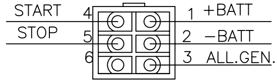
VISTA LATO INSERIMENTO CAVI
