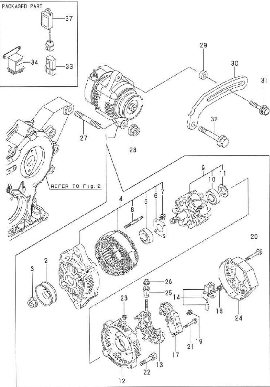
Fig.14.GENERATOR
